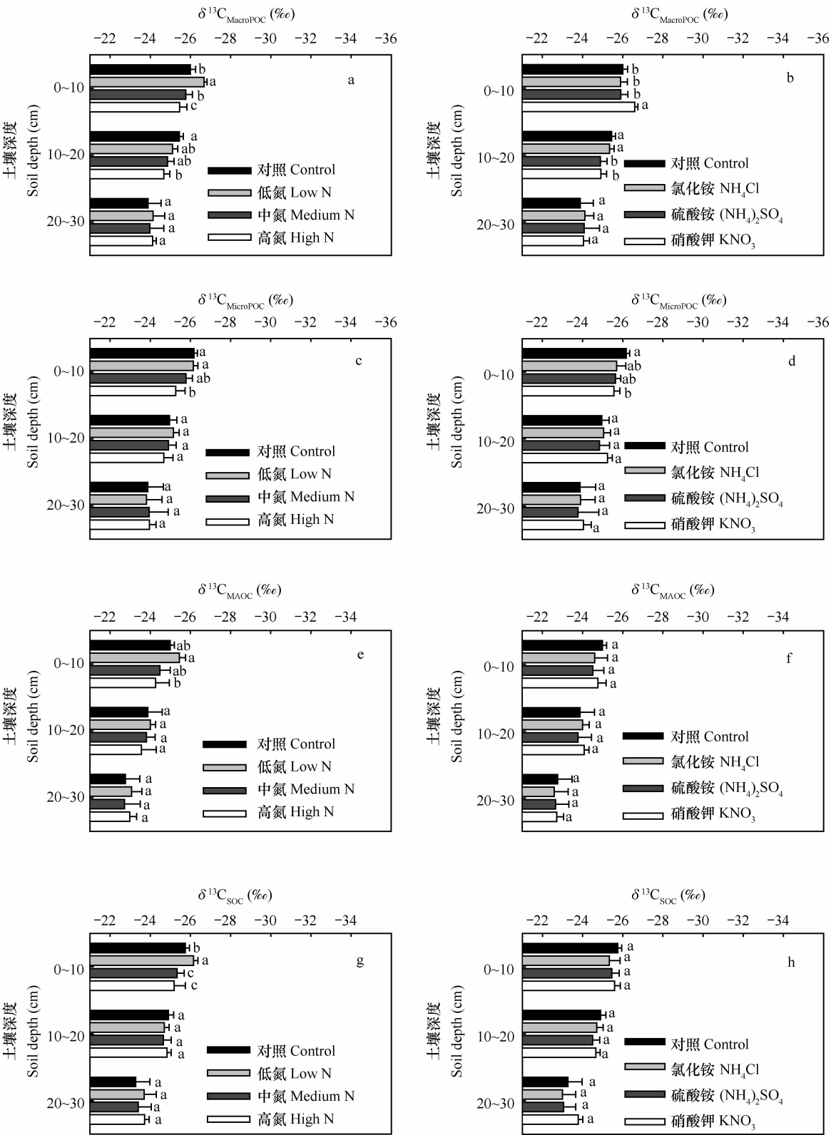
图3 不同施氮剂量和施氮类型下总SOC以及三个组分 \delta^{13}\text{C} 值的变化 (图中不同字母表示同层土壤各处理差异显著)
