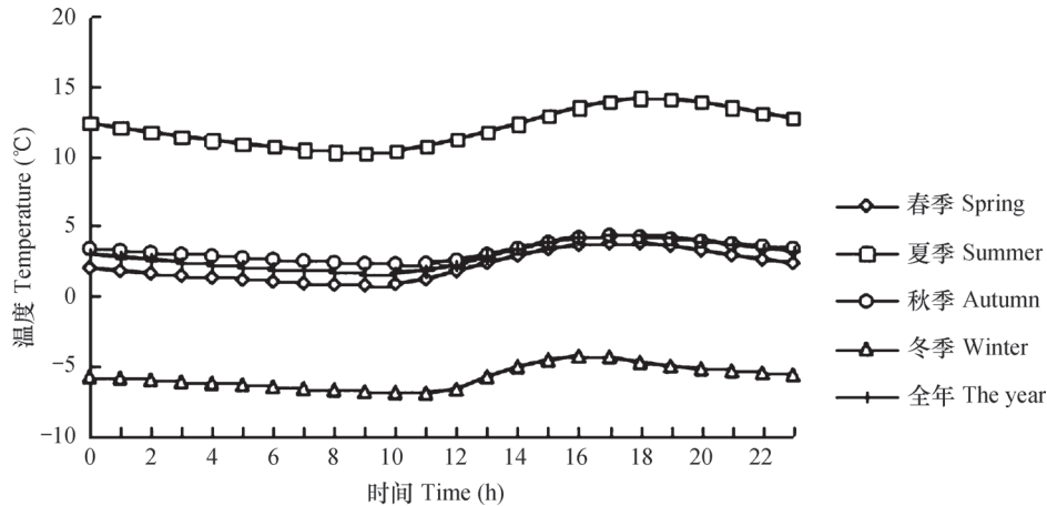
图3 四季及全年土壤温度的日变化
