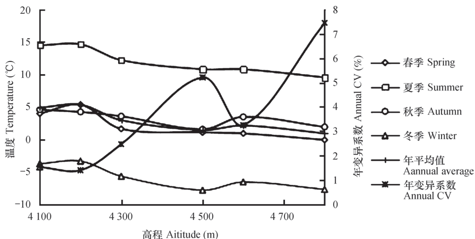
图4 土壤温度及变异系数与海拔梯度之间关系
