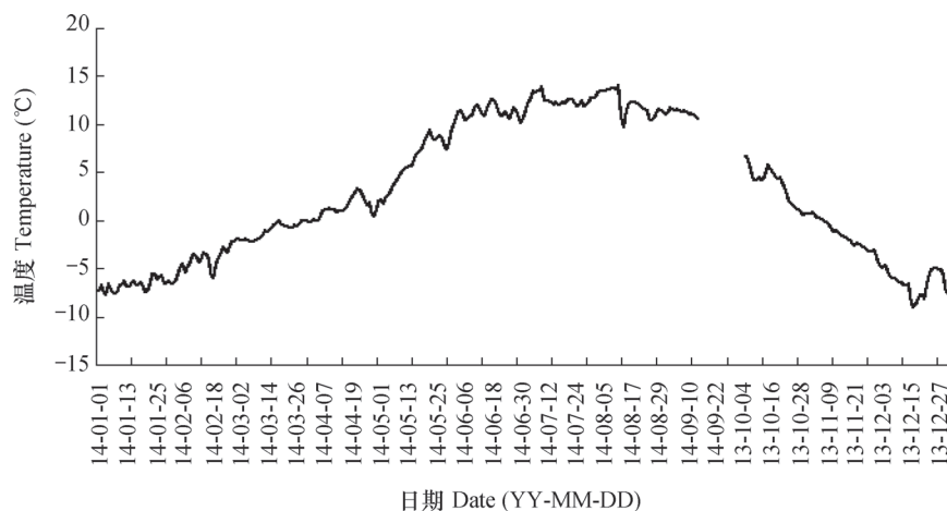
图2 土壤日平均温度年内变化
