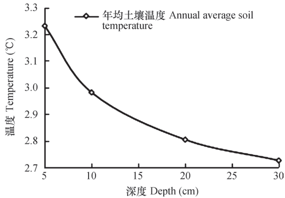
图5 不同深度土壤温度年平均变化特征
