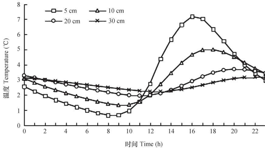
图6 不同深度土壤温度日变化过程
