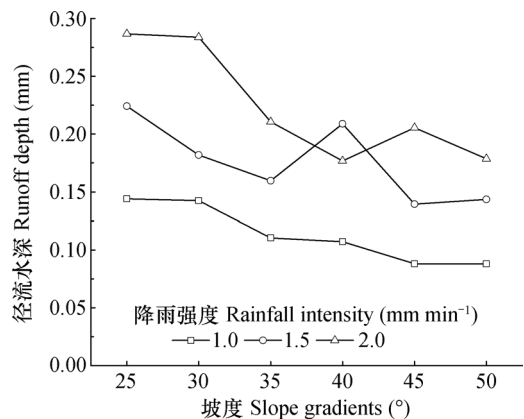
图2 平均径流水深随雨强和坡度的变化
