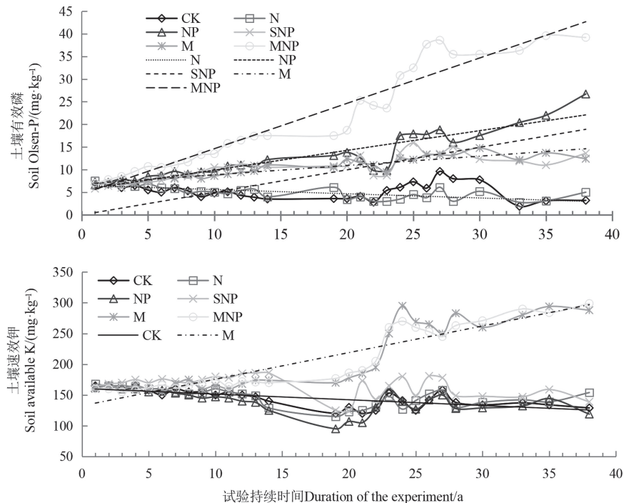
图4 施肥对土壤有效磷和速效钾贡献
