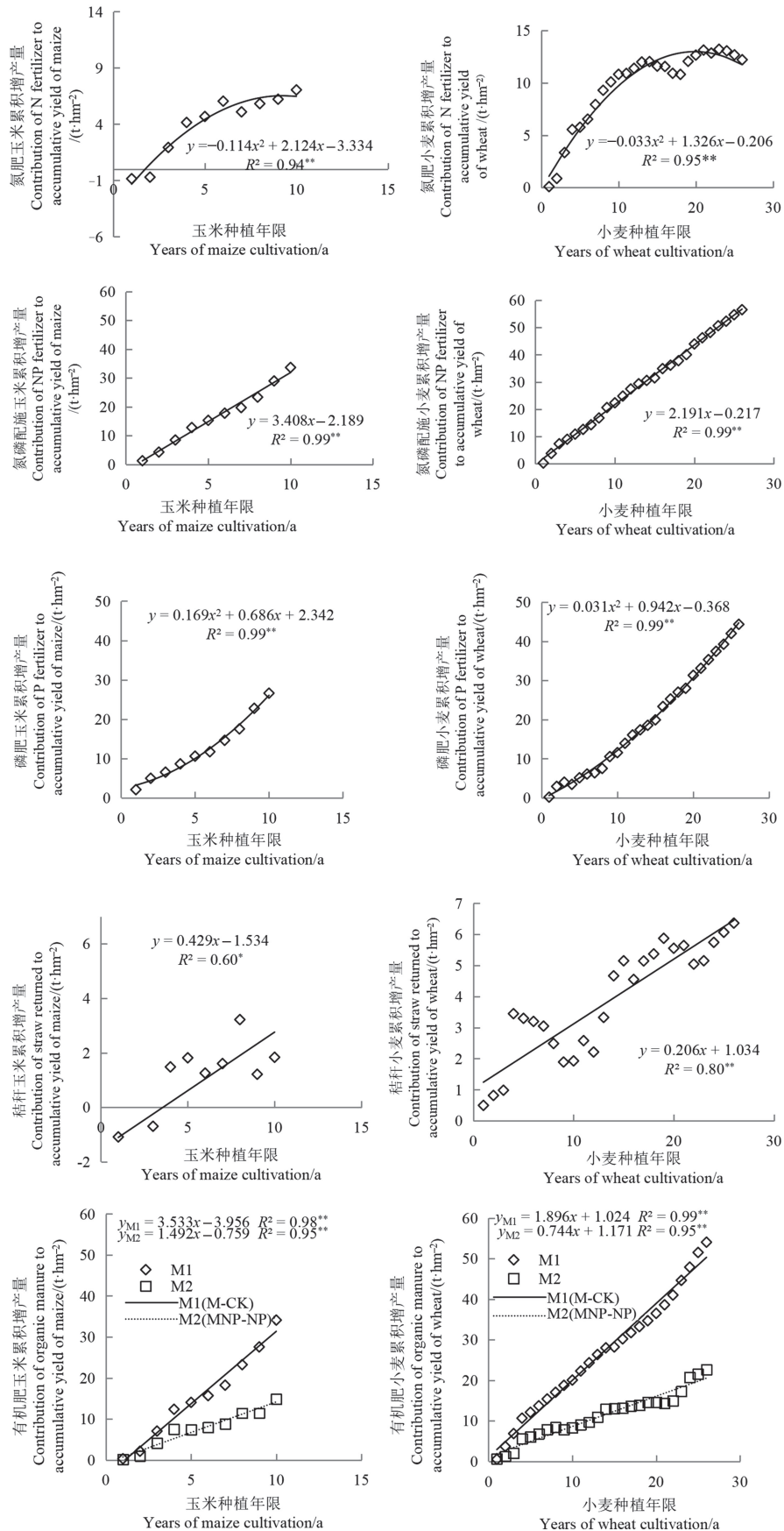
图2 不同施肥处理小麦和玉米累积增产产量
