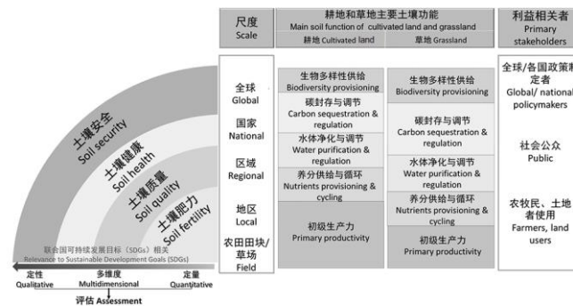
图 2 “土壤健康” 相关概念内涵之间关系图 (据 Lehmann 等 [16] 修改)
