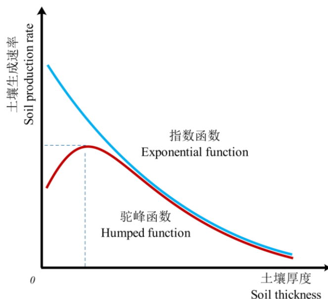
图 2 土壤生成速率随土壤厚度变化函数 [16]
