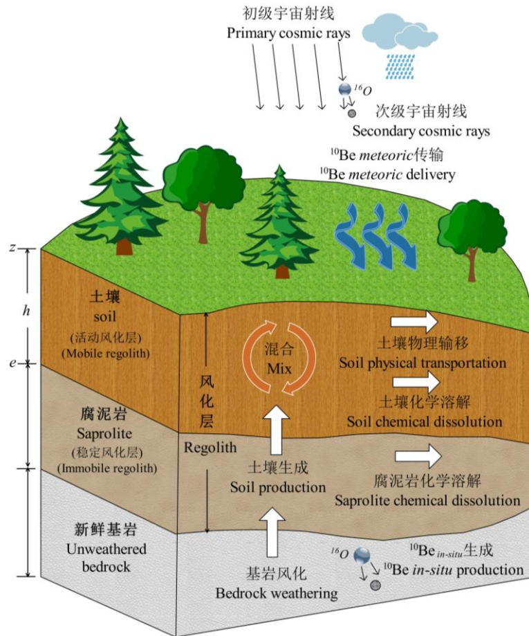
图 1 山坡风化层剖面演化过程 [15]
