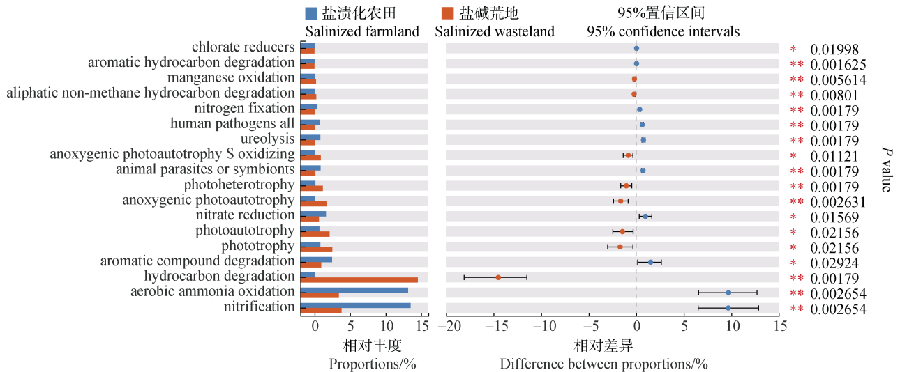
图 7 基于 FAPROTAX 预测的两种土地利用类型盐渍化土壤原核生物潜在功能差异
