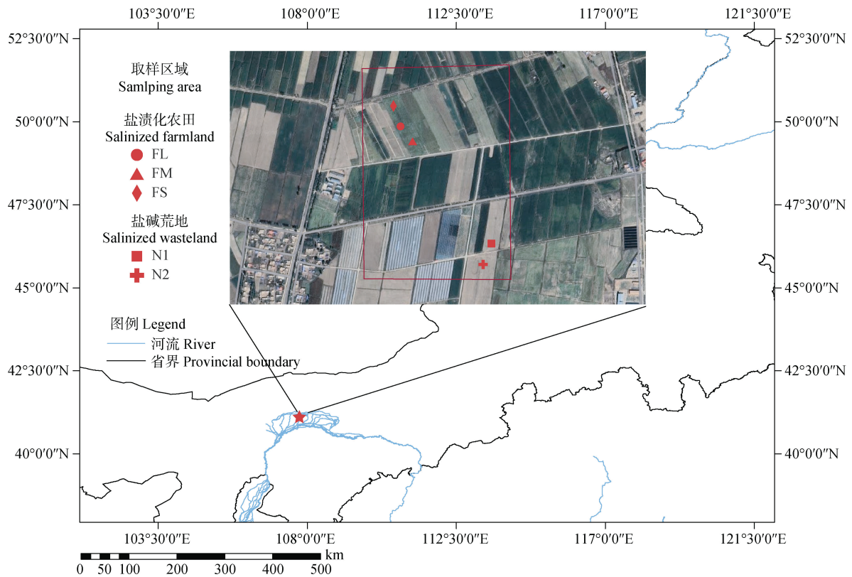
图 1 土壤样品采集区域
