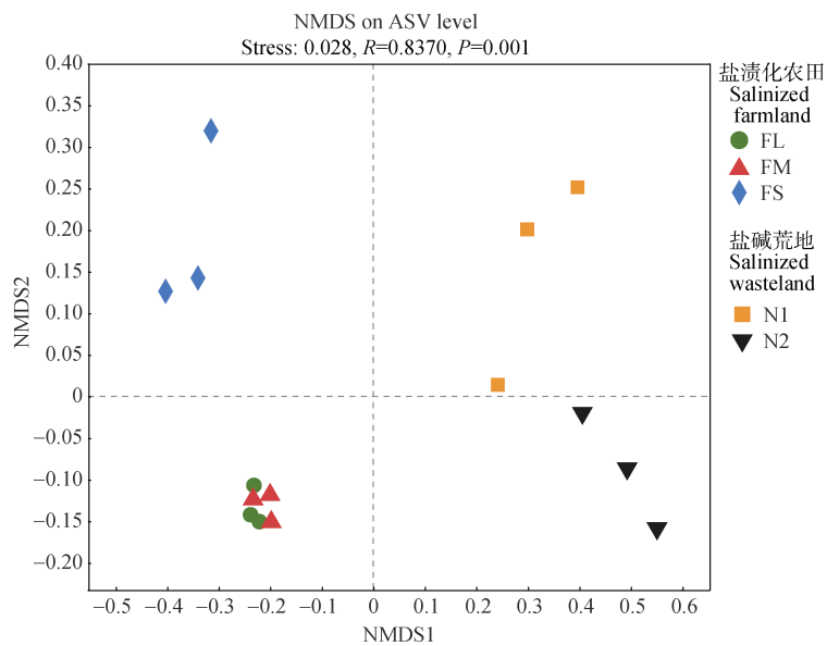
图 4 不同土地利用类型下盐渍化土壤原核生物 β 多样性 NMDS 分析
