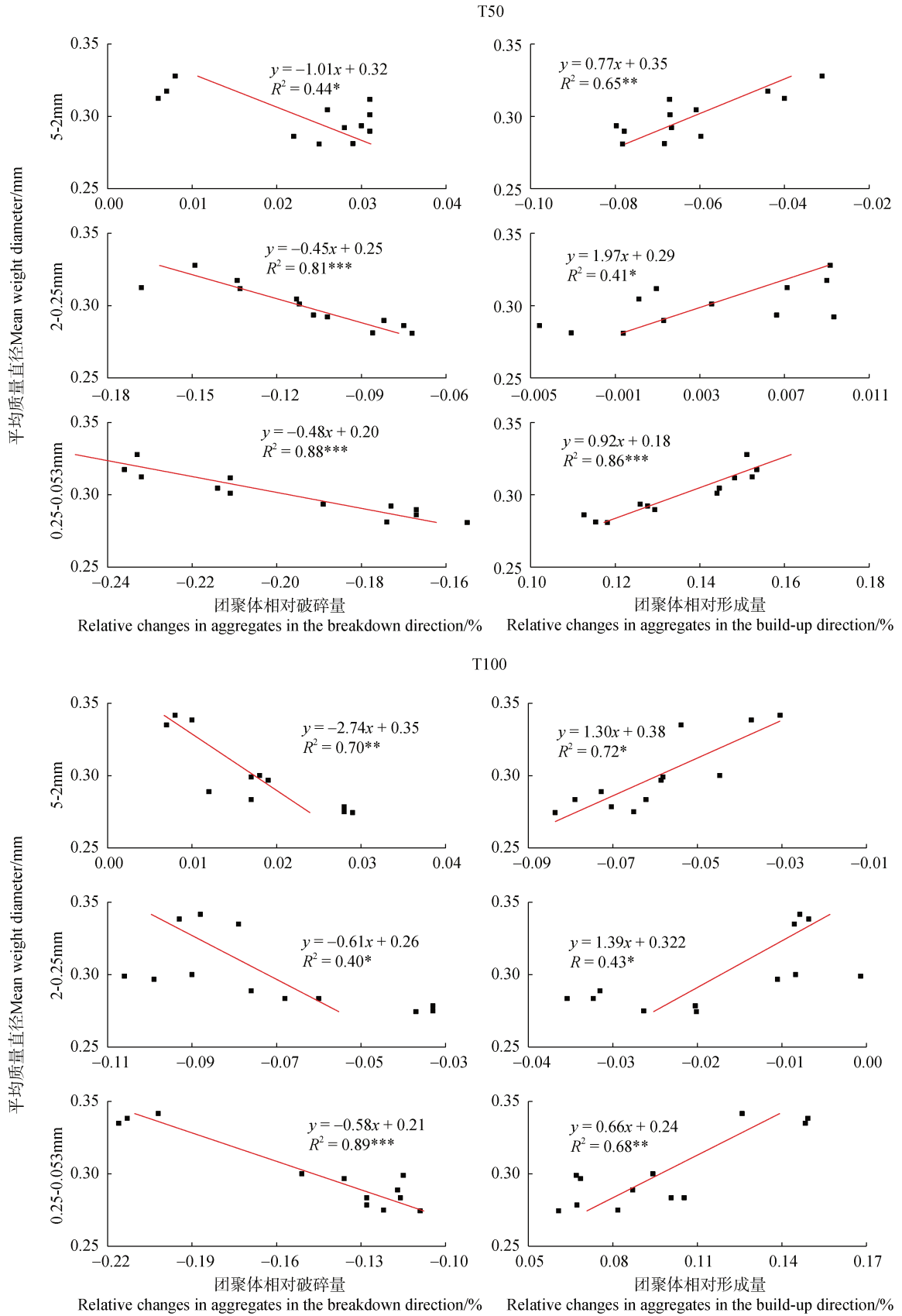
图 5 不同处理下平均质量直径与团聚体相对变化量的关系
