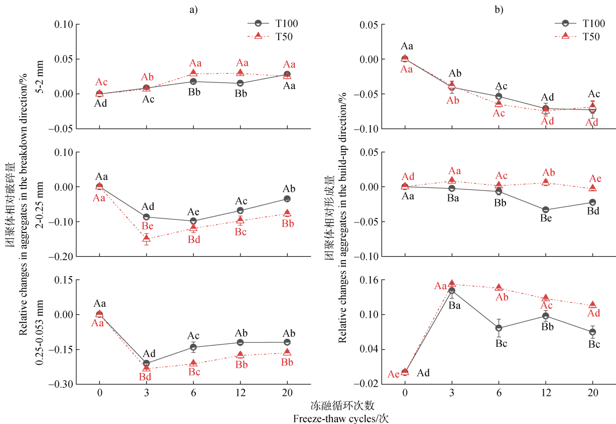
图 4 不同处理下土壤团聚体相对破碎 (a) 和形成量 (b)
