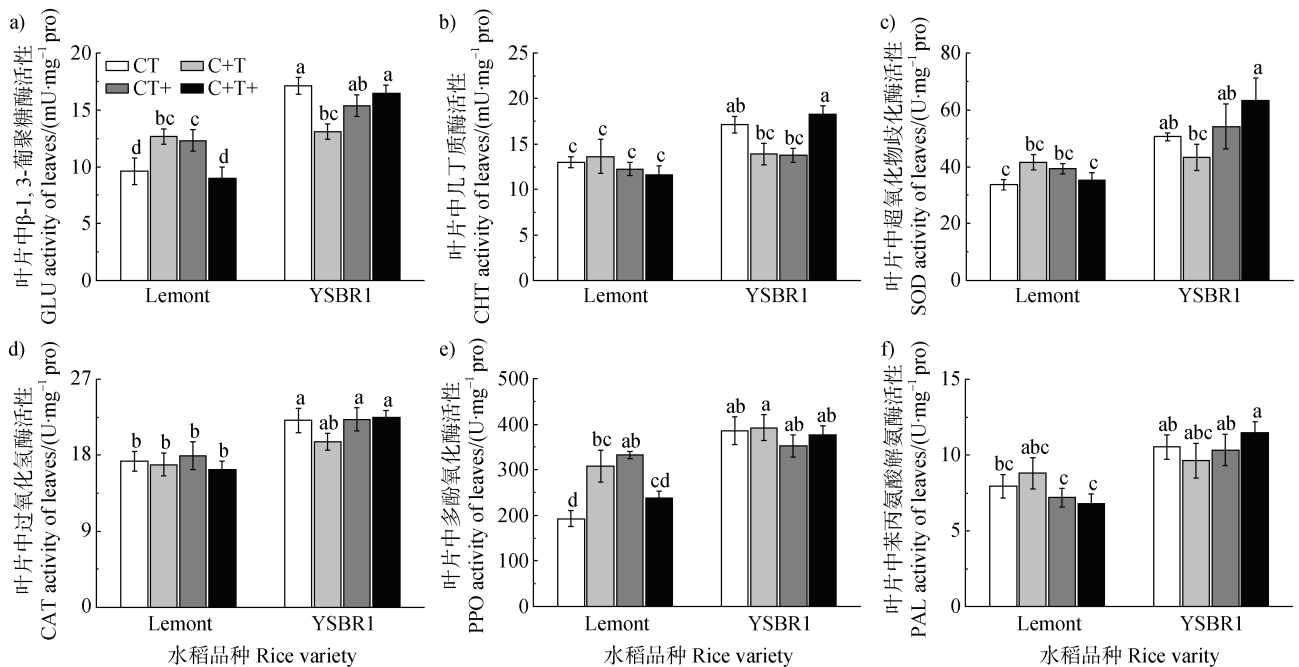
图 2 不同[CO 2 ]和温度处理对感病后的 Lemont 和 YSBR1 叶片中 β-1, 3-葡聚糖酶 (a)、几丁质酶 (b)、超氧化物歧化酶 (c)、过氧化氢酶 (d)、多酚氧化酶 (e) 和苯丙氨酸解氨酶 (f) 活性的影响
