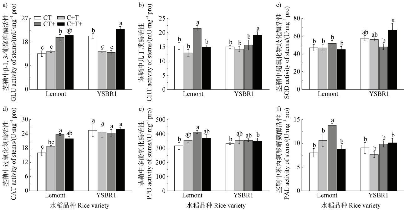
图 3 不同[CO 2 ]和温度处理对感病后的 Lemont 和 YSBR1 茎鞘中 β-1, 3-葡聚糖酶 (a)、几丁质酶 (b)、超氧化物歧化酶 (c)、过氧化氢酶 (d)、多酚氧化酶 (e) 和苯丙氨酸解氨酶 (f) 活性的影响
