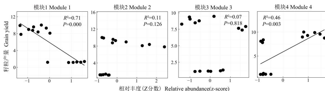
图 6 不同施肥处理模块相对丰度与小麦产量的回归分析
