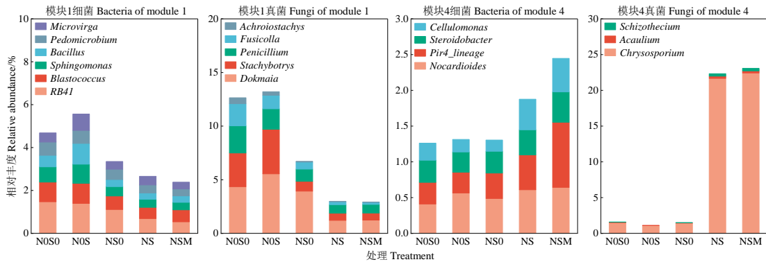
图 7 不同施肥处理模块优势属
