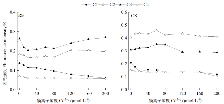
图 6 稻虾种养(RS)和水稻单作(CK)系统土壤 DOM 各组分与 Cd 2+ 猝灭反应的荧光强度变化
