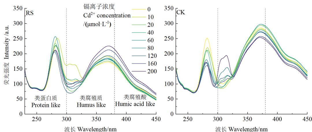
图 4 稻虾种养(RS)和水稻单作(CK)系统土壤 DOM 与 Cd^{2+} 猝灭反应的同步荧光光谱
