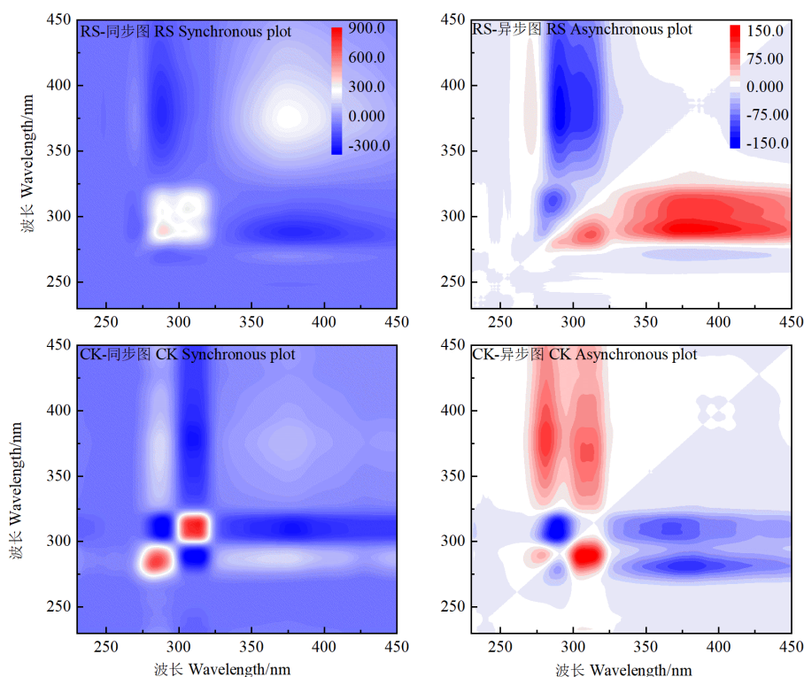
图 5 稻虾种养(RS)和水稻单作(CK)系统土壤 DOM 与 \text{Cd}^{2+} 猝灭反应的同步和异步图
