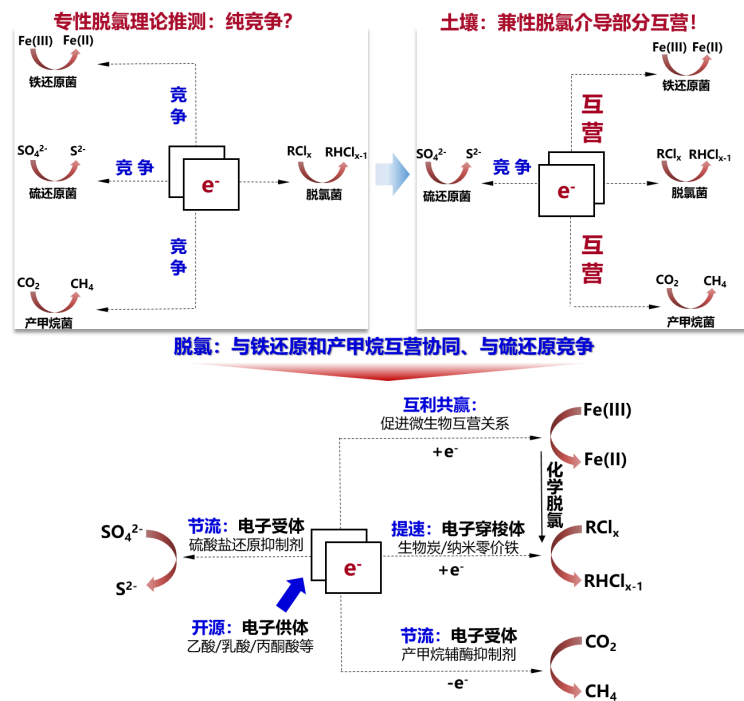
图 2 基于电子分流干预的土壤 OCPs 污染多过程协同靶向调控方法原理
