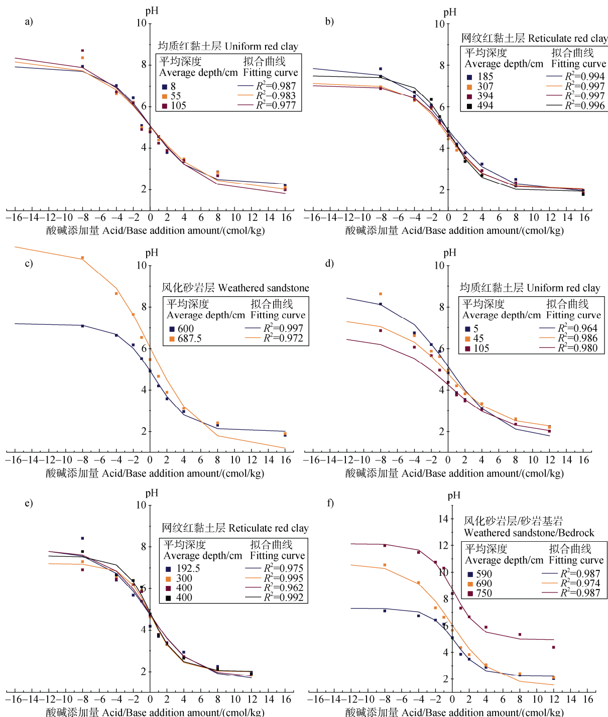
图 1 BH5 (a, b, c) 和 BH8 (d, e, f) 钻孔点红壤风化壳不同深度样品的酸碱滴定曲线
