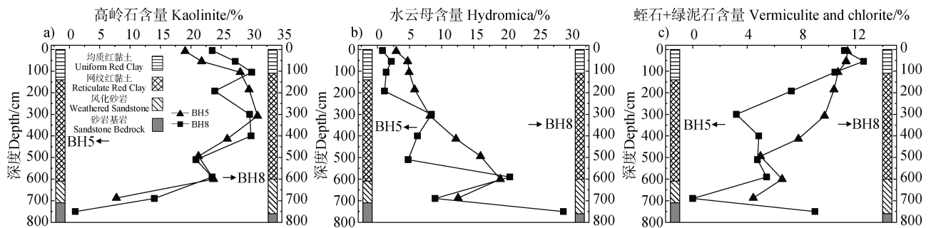
图 7 BH5 和 BH8 钻孔点红壤风化壳矿物组成的深度变化特征
