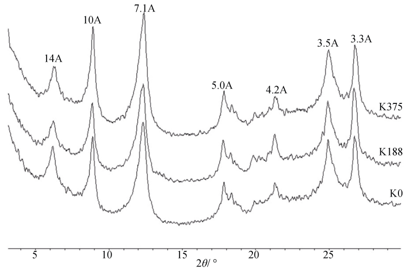
图 2 不同施肥处理土壤黏粒矿物 X-射线衍射 (XRD) 图谱比较
