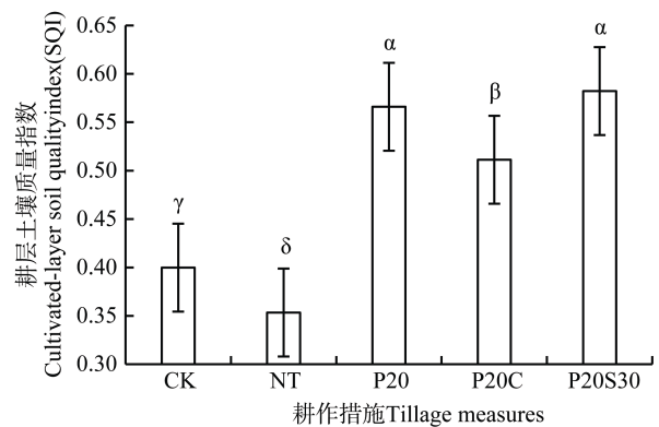
图 6 不同耕作措施下坡耕地耕层土壤质量指数变化
