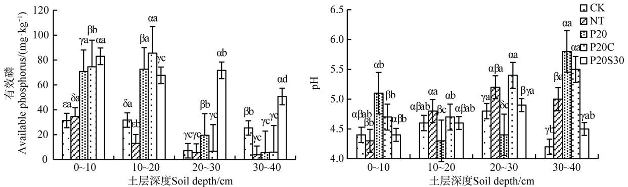
图4 不同耕作措施下坡耕地土壤有效磷和 pH 变化特征
