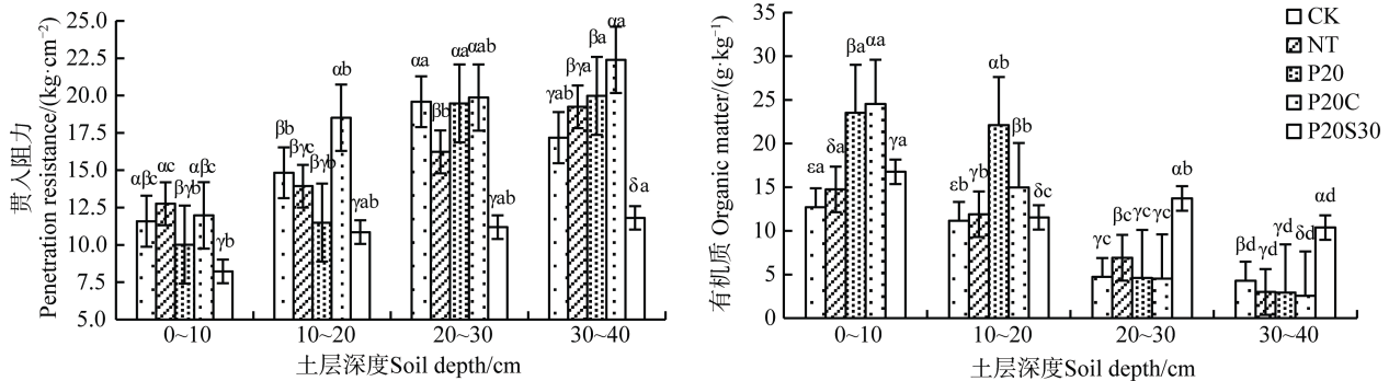
图3 不同耕作措施下坡耕地土壤贯入阻力和有机质变化特征
