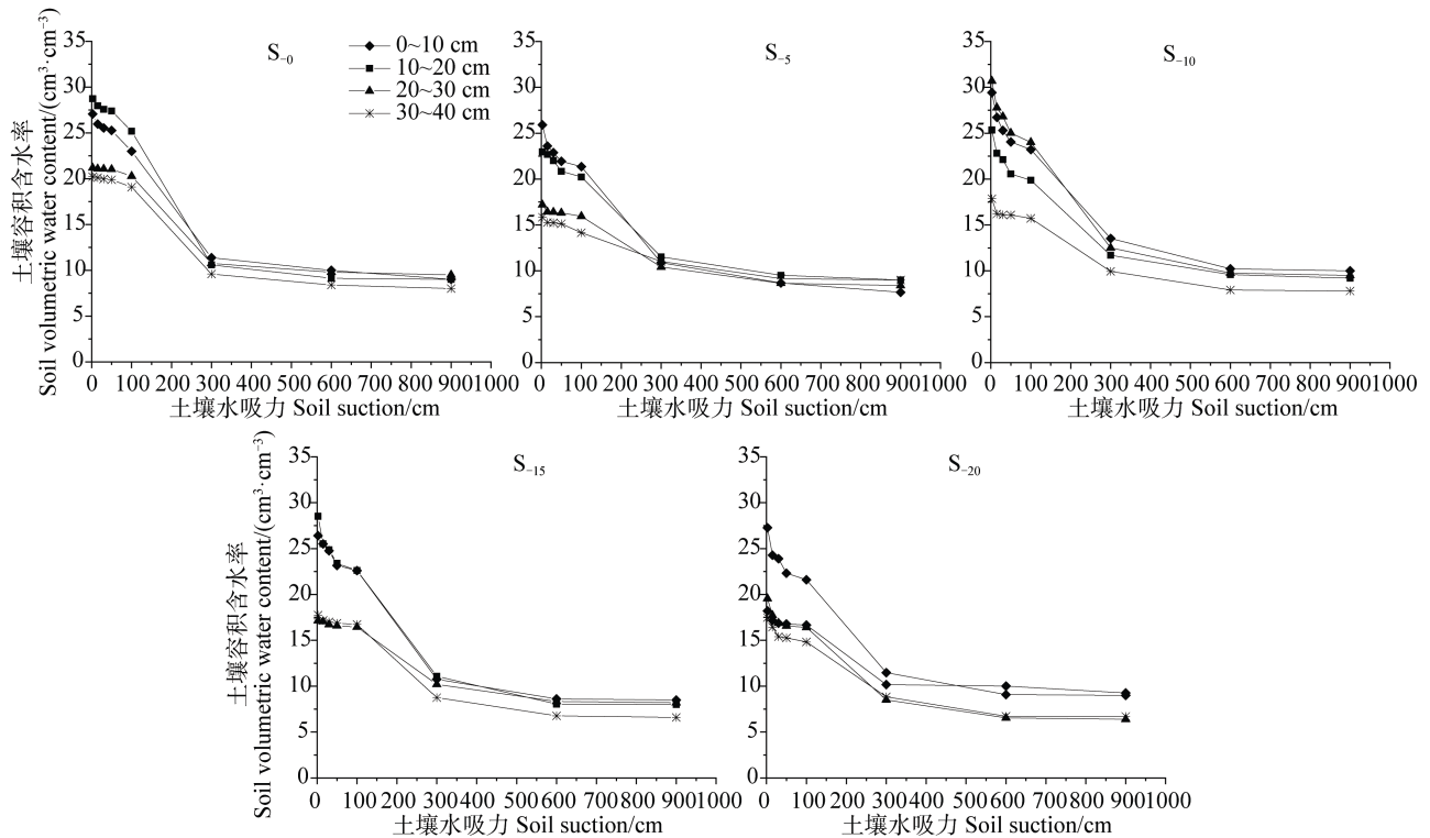
图 1 不同侵蚀程度坡耕地土壤容积含水率变化
