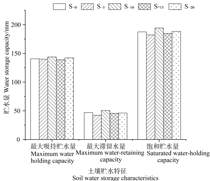
图3 不同侵蚀程度坡耕地0~40 cm土壤贮水特征
