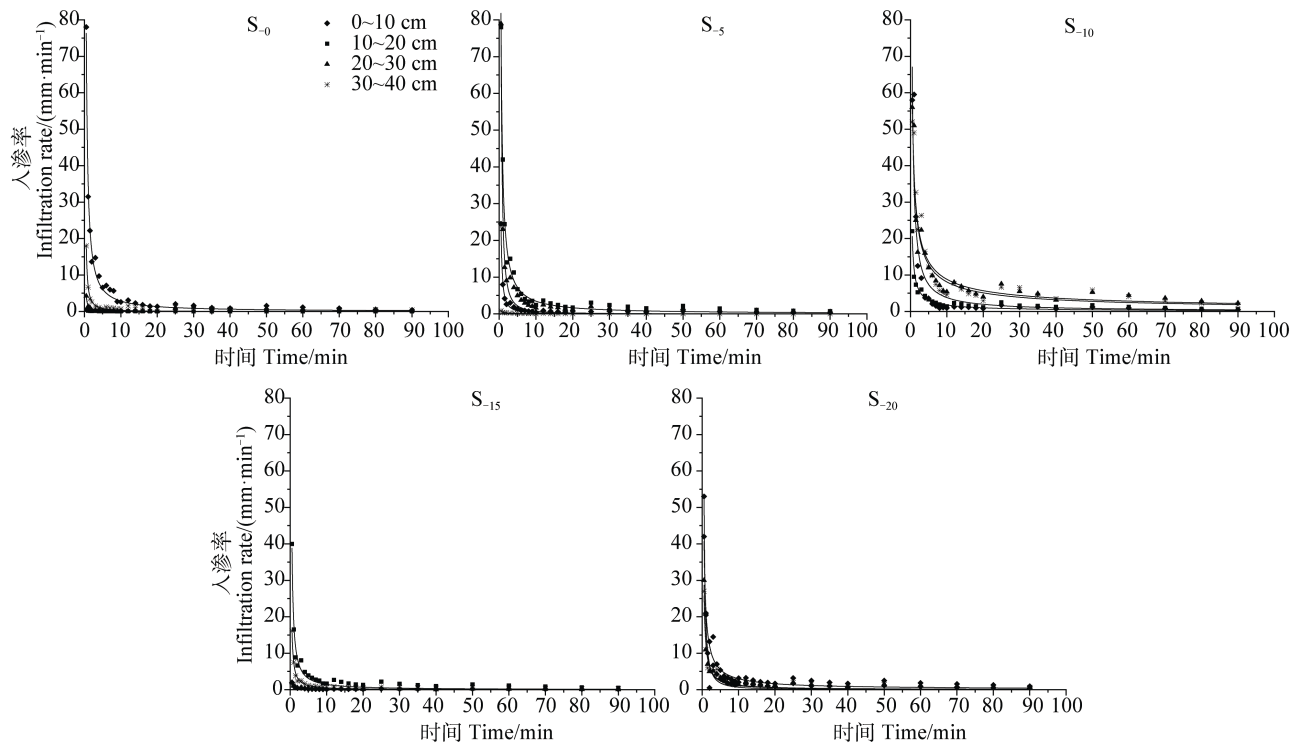
图2 不同侵蚀程度坡耕地土壤入渗特征
