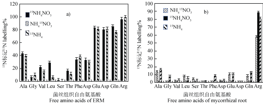
图 1 AM 真菌共生系统中菌丝室用 ^{15}\text{NH}_4\text{NO}_3 或 \text{NH}_4^{15}\text{NO}_3 处理 6 天时其根外菌丝 (a) 和菌根组织 (b) 自由氨基酸的 ^{15}\text{N} 标记
