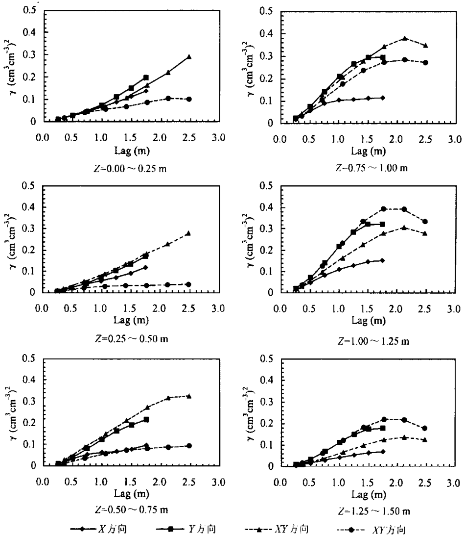
图2 三维空间上的土壤含水量分布在四个方向上的实验半变差图(测量时间为1997年4月2日19:00)
