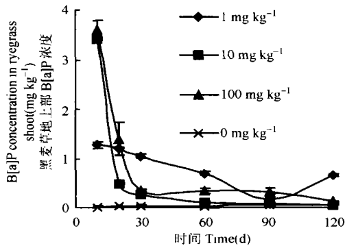
图3 黑麦草地上部中苯并[a]芘浓度的动态变化
