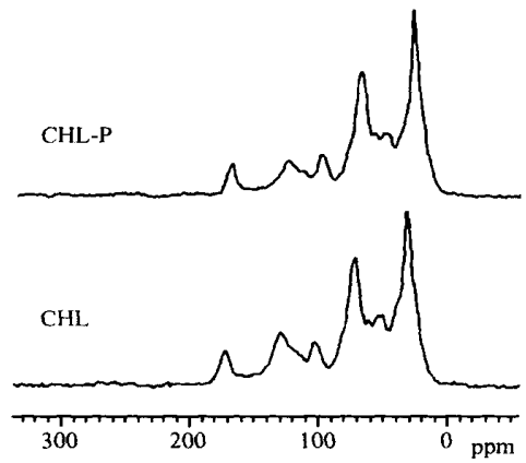
图1 CHL和CHL-P土壤的 13 C CP-MAS NMR图
