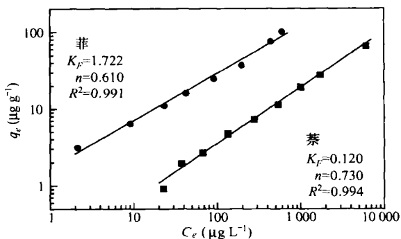
图 2 菲和萘在 GZ1 土壤上的吸附等温线
