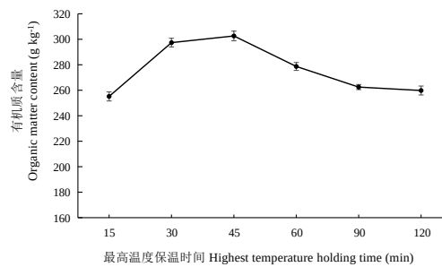
图 3 最高温度保温时间对鸡粪有机质含量的影响
