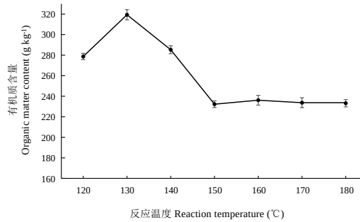
图 2 反应温度对鸡粪有机质含量的影响
