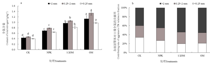
图 2 土壤团聚体中全氮含量 (a) 及其对土壤全氮的贡献率 (b)
