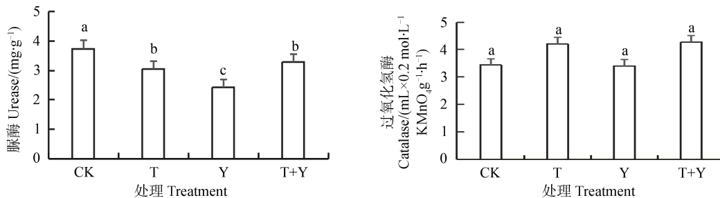
图 2 硒处理下土壤脲酶和过氧化氢酶活性
