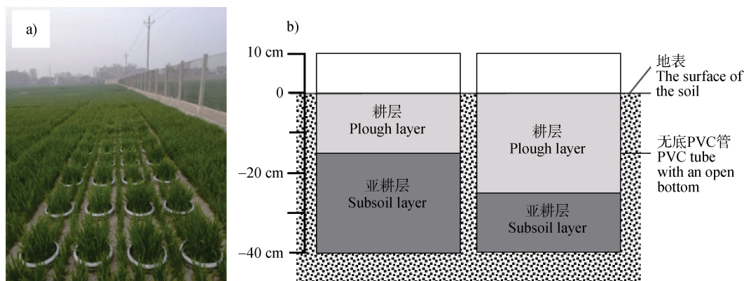
图 1 土柱田间排列 (a) 及不同耕层厚度处理实验设计 (b) 示意图
