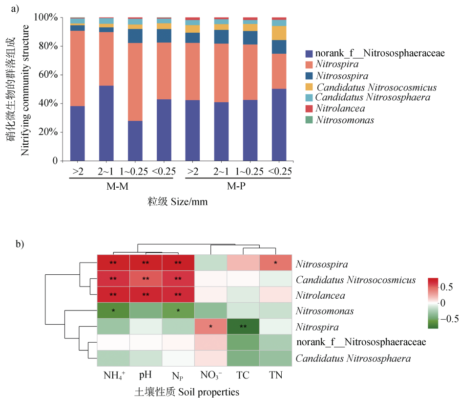
图 4 基于 16S rRNA 基因的硝化微生物群落组成 (a) 及与土壤性质和硝化潜能的相关系数热图分析 (b)
