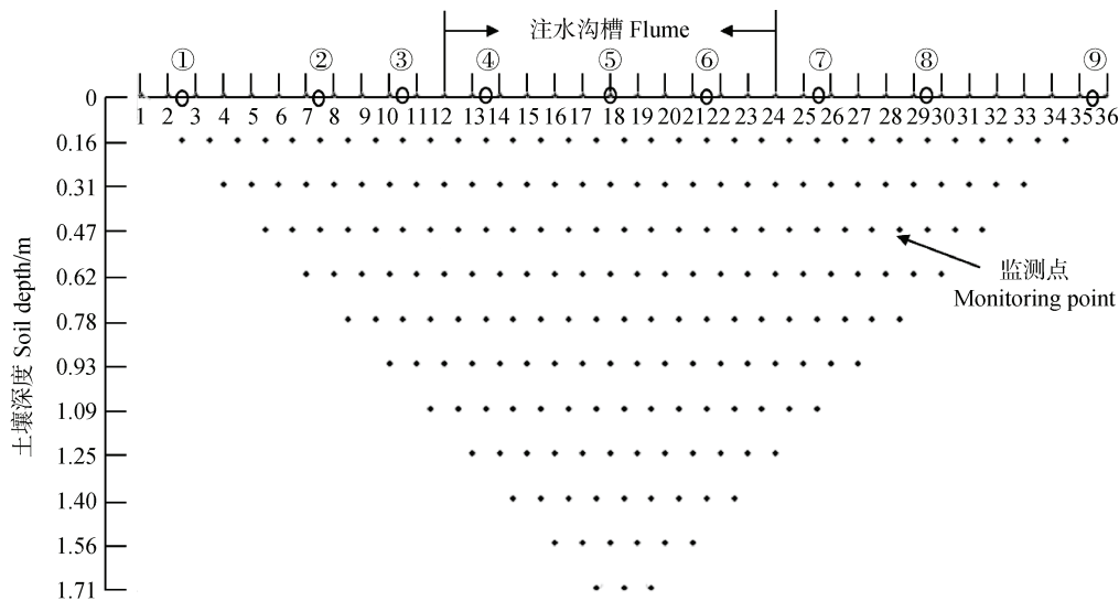
图 2 电阻率层析成像测量点位图
