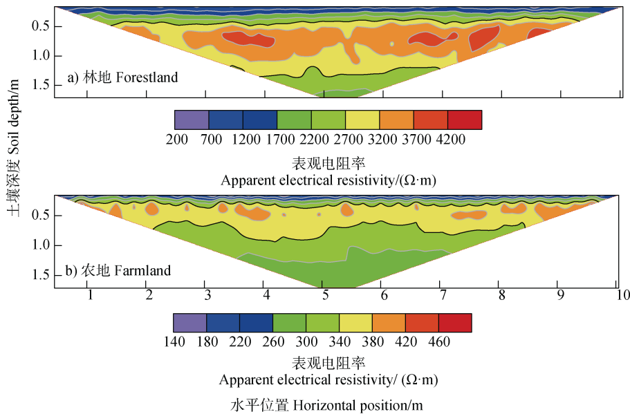
图 3 两种土地利用类型土壤表观电阻率初始值的剖面分布
