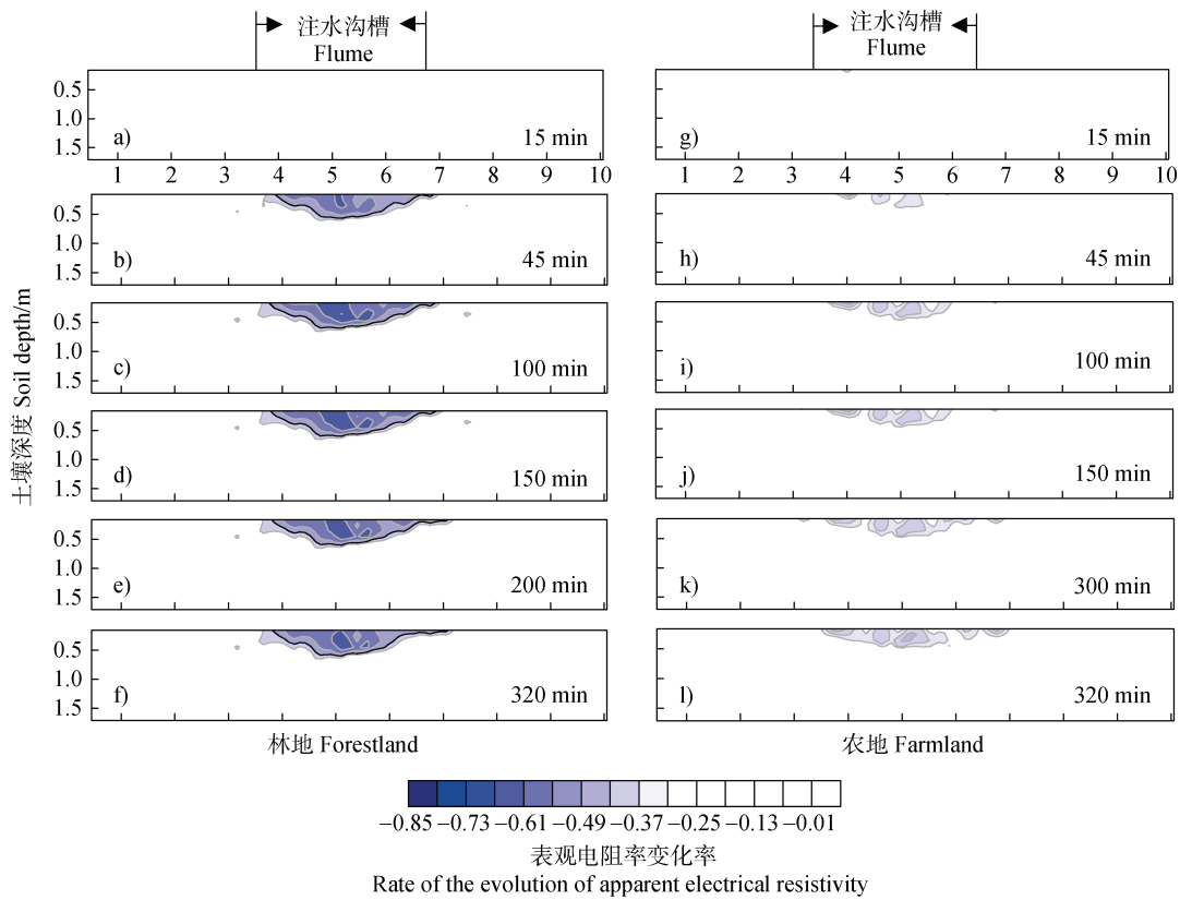
图 4 第一阶段（注水 100 L）土壤剖面表观电阻率变化率动态
