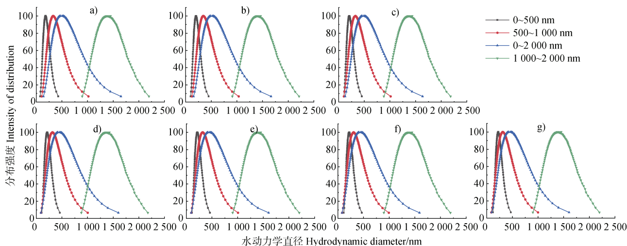
图 1 土壤 (a. 黑土; b. 暗棕壤; c. 黄棕壤; d. 黄壤; e. 红壤; f. 赤红壤; g. 砖红壤) 颗粒的水动力直径分布
