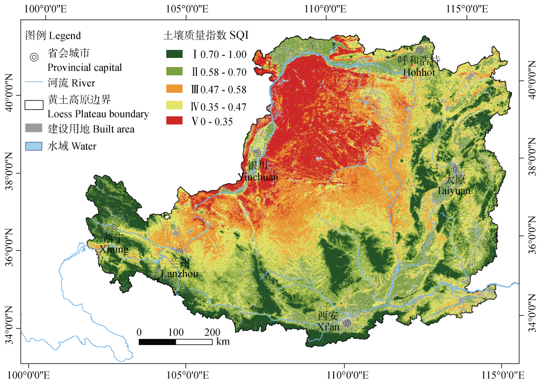
图 1 黄土高原土壤质量空间分布 Fig. 1 Spatial distribution of soil quality in the Loess Plateau
