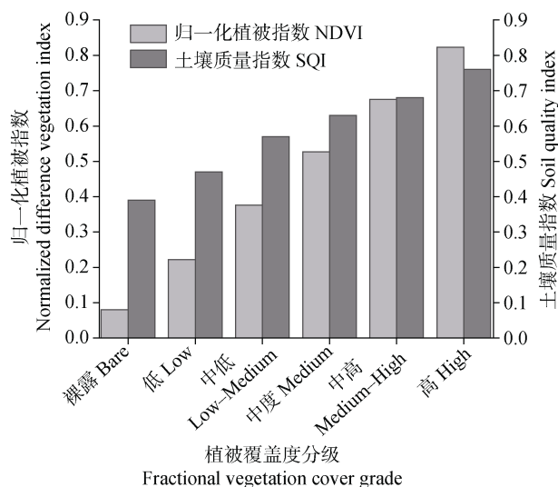
图2 不同植被覆盖度下NDVI和土壤质量的关系
