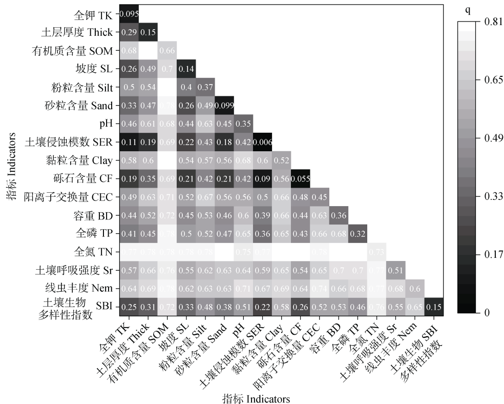
图 5 土壤质量影响因子交互作用强度结果
