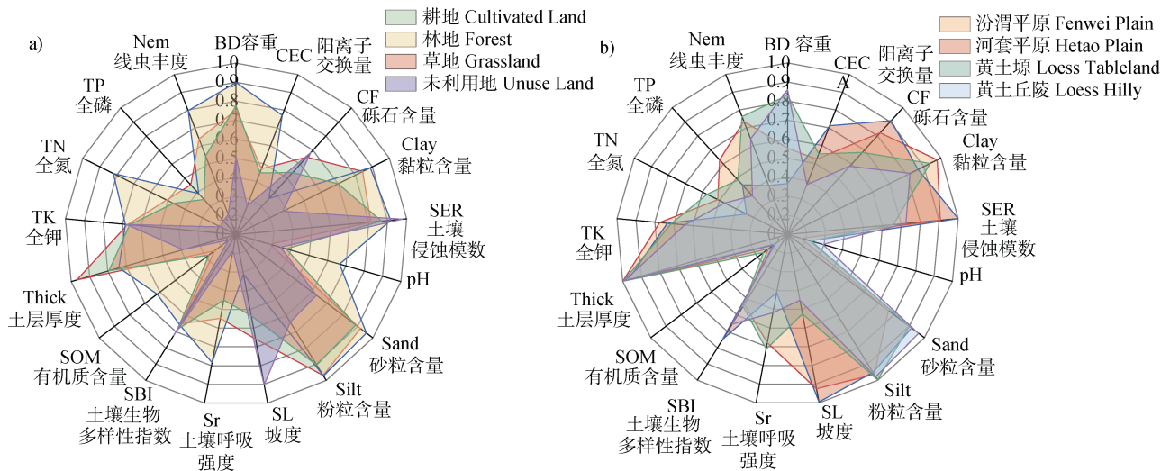
图 6 不同土地利用类型 a) 和农业区耕地 b) 土壤质量评价指标得分
