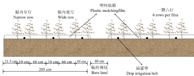
图 2 种植模式图
