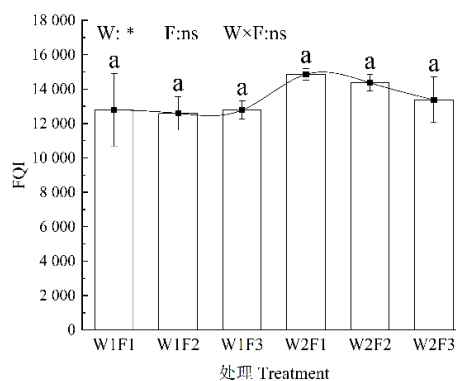
图 7 不同处理对棉纤维品质指数 (FQI) 的影响
