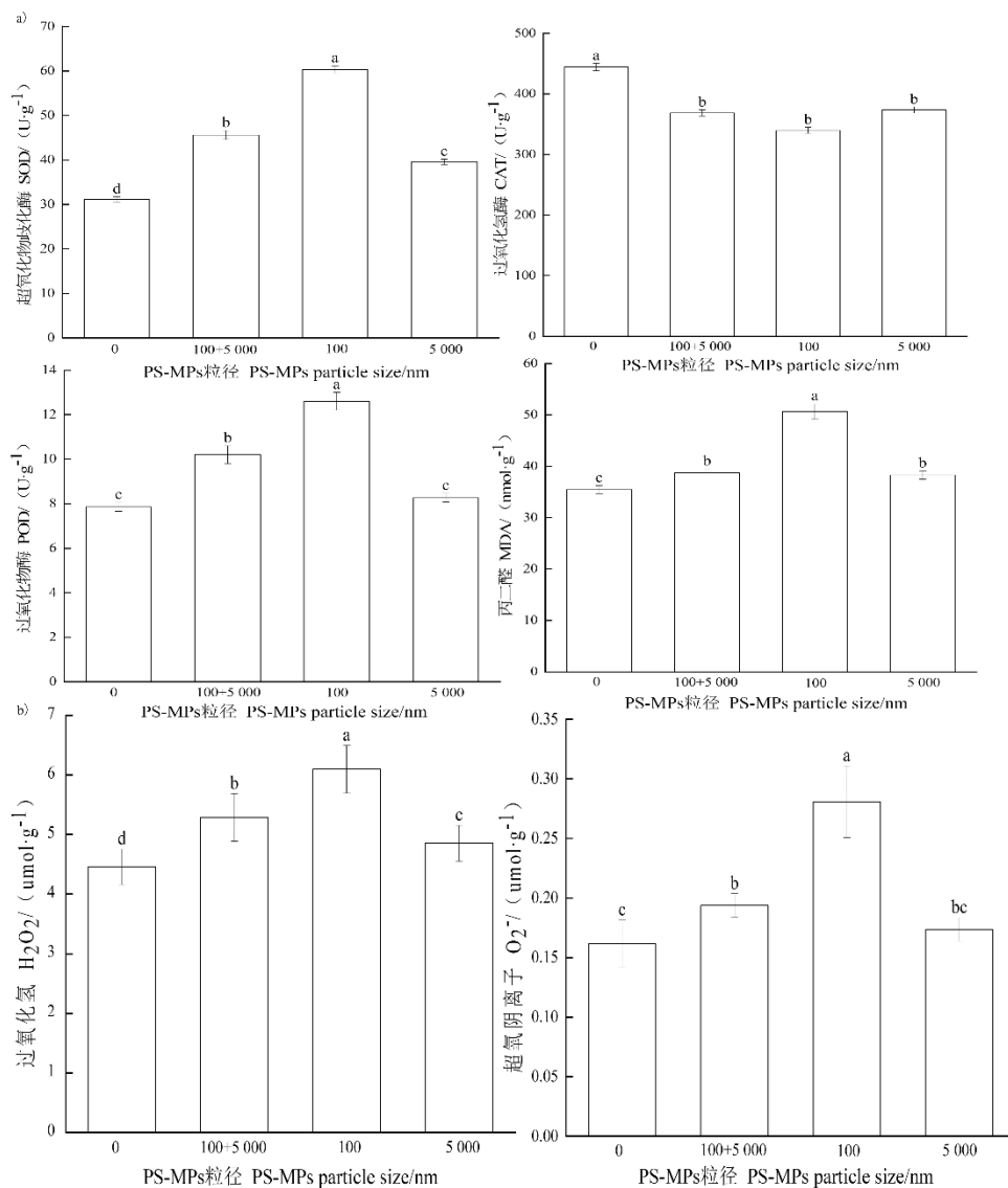
图 4 多粒径 PS-MPs (0、100+5 000、100、5 000 nm) 暴露对玉米幼苗 SOD、CAT、POD 活性与 MDA 含量的影响 (a) 和过氧化氢 (H 2 O 2 ) 与超氧阴离子 (O 2 - ) 积累水平的影响 (b)
