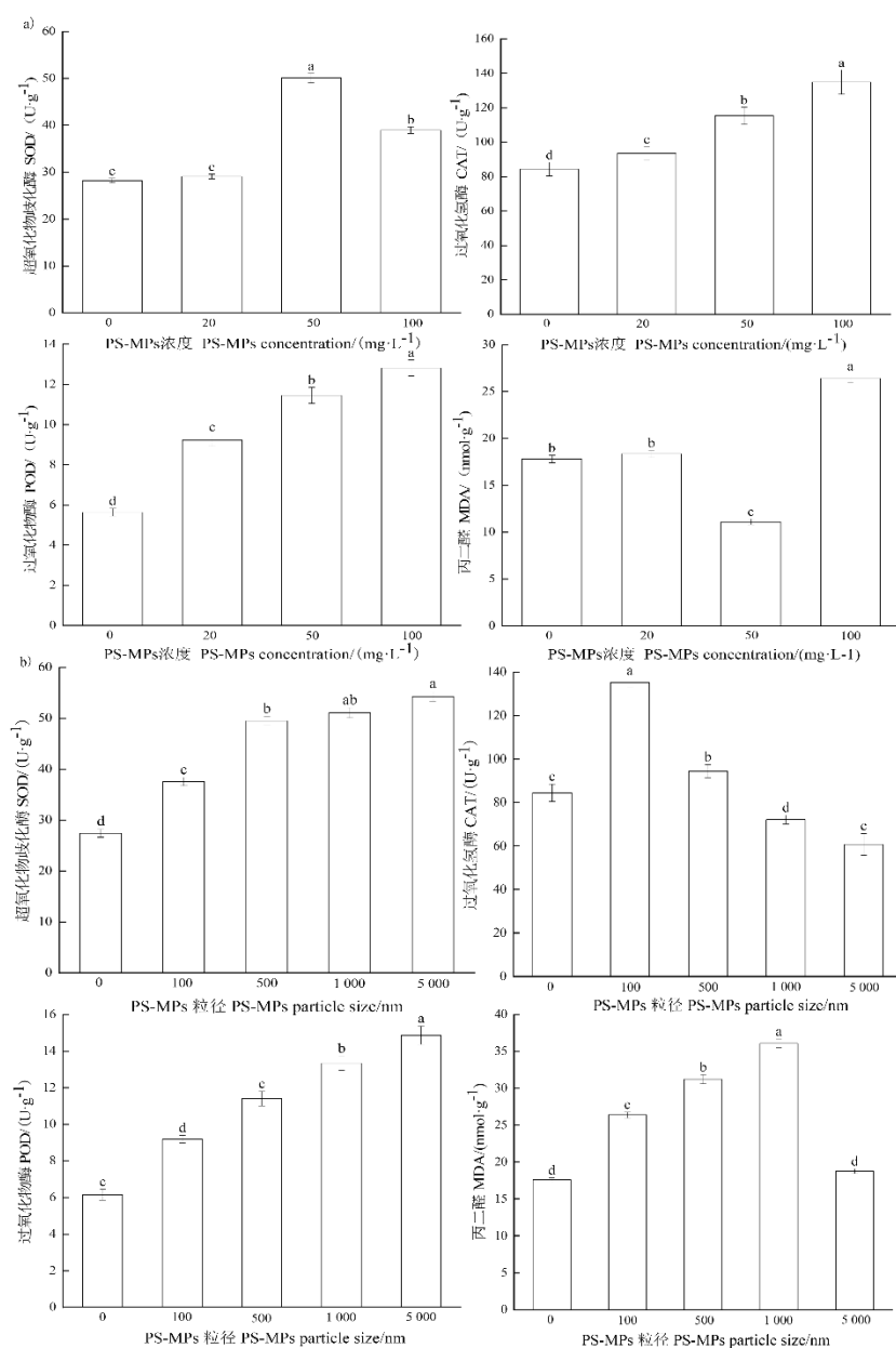
图 3 不同浓度 PS-MPs (0、20、50、100 mg·L -1 ) (a) 和不同粒径 PS-MPs (0、100、500、1 000 和 5 000
